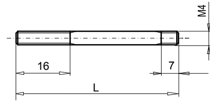
TIRANT M4xL
