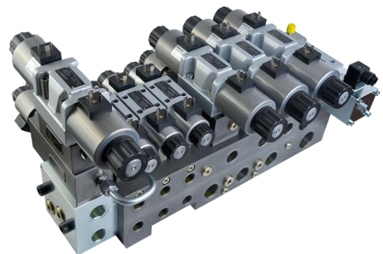
Kundenspezifische Steuereinheit
